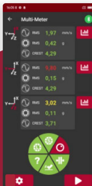
MODO MULTIMETRO
